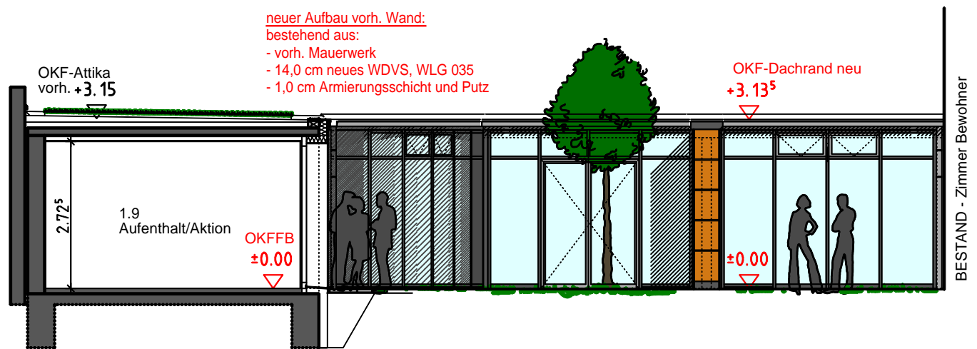
Schnitt B-B
